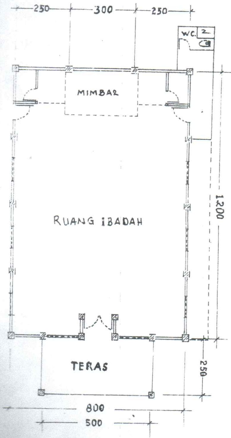
DENAH SKALA 1 : 100
